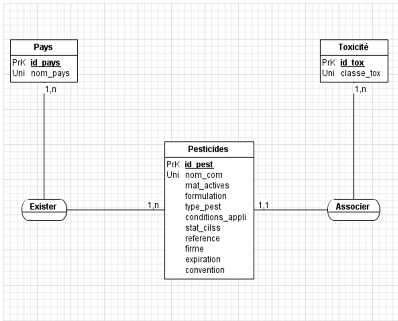
Figure 1 : Schéma du modèle conceptuel des données
